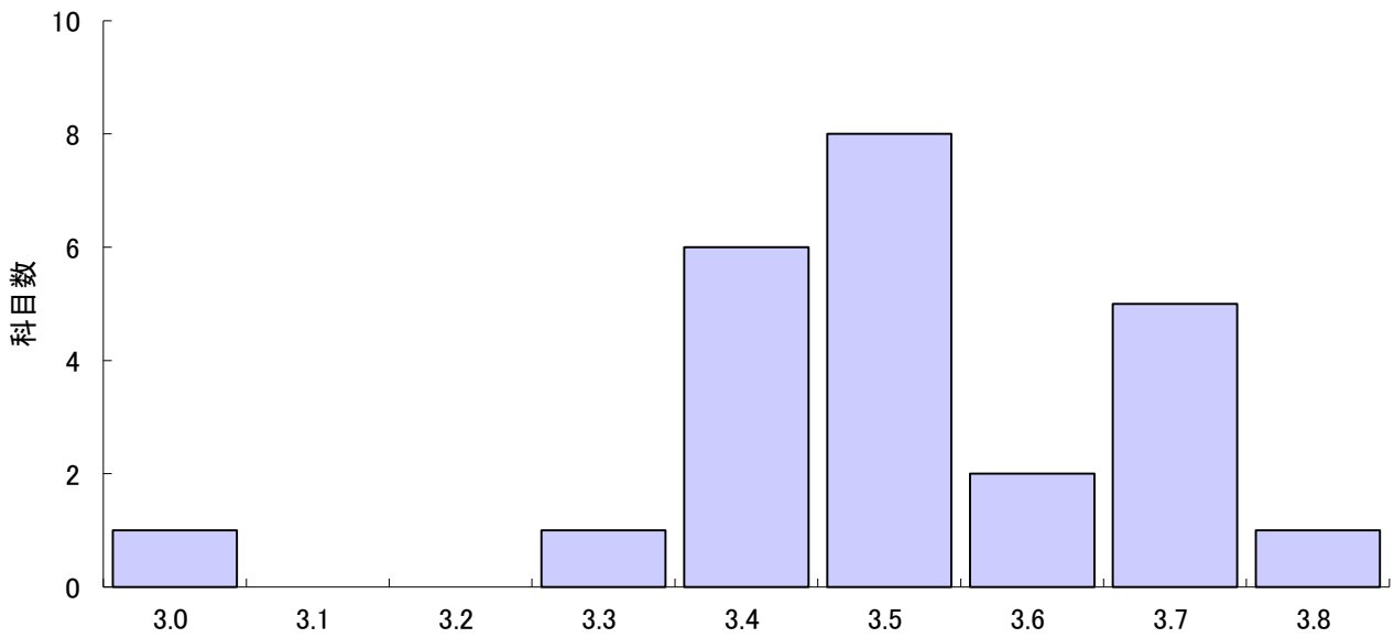
Fig.3 平均点別度数分布
